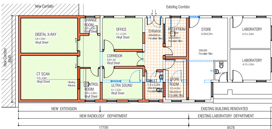
Grundrissplan neuer Radiologie Trakt
